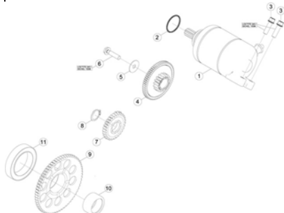
TAV.07 Avviamento elettrico - Electric starter - Dé marrage électrique - Elektrischer start - Arranque elétrico
