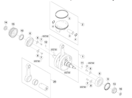
TAV.02A Albero motore - Crankshaft - Vilebrequin - Kurbelwelle - Cigüeñal
