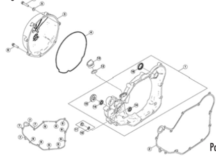
TAV.01A Coperchio frizione - Clutch cover - Couverde d'embrague - Kupplungsdeckel - Tapa embrague
