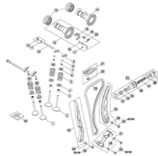
TAV.11A Valvole-Catena distribuzione - Valves-Timing chain - Soupapes-Chaîne de distribution - Ventil-Steuerkette - Válvulas-Cadena de distribución
